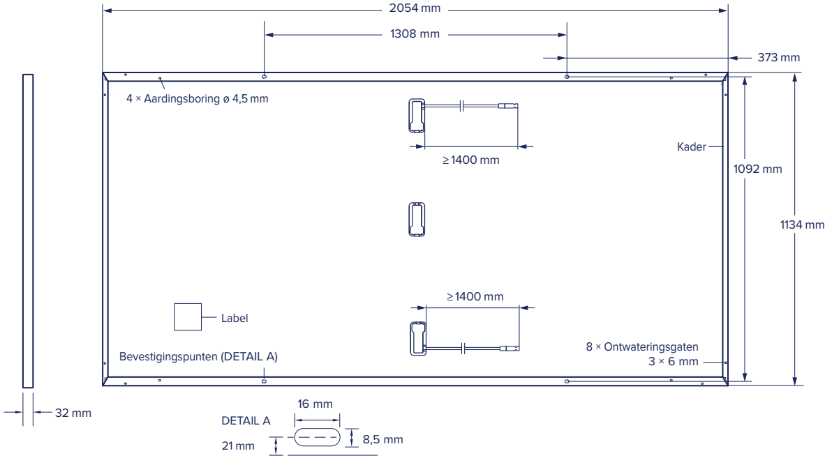
Afb. 1: Buitenafmetingen (in mm) en componenten voor Q.PEAK DUO ML-G11.2.
