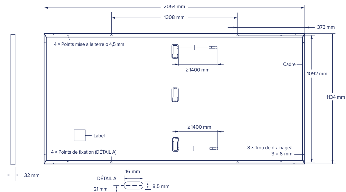
Fig. 1: Dimensions externes (en mm) et composants pour Q.PEAK DUO ML-G11.2.
